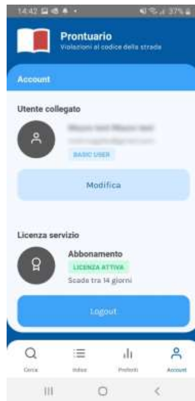
Figura 4. Info licenza
