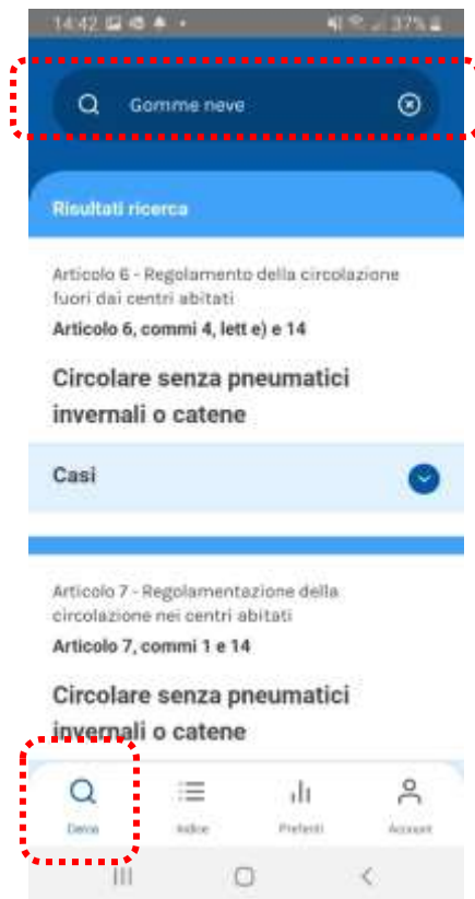
Figura 5. Ricerca avanzata
